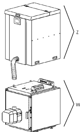
Rysunek 3. Modułowa budowa kotła
