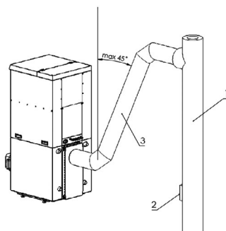
Rysunek 14. Podłączenie do instalacji kominowej – proste 1 – Przewód kominowy; 2 – Wyczystka kominu; 3 – Zaizolowane podłączenie do kominu.
