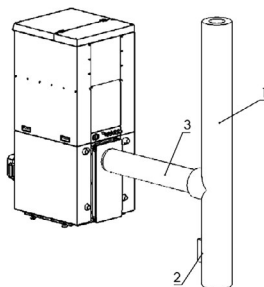
Rysunek 15. Podłączenie do instalacji kominowej – pochylone 1 – Przewód kominowy; 2 – Wyczystka kominu; 3 – Zaizolowane podłączenie do kominu.
